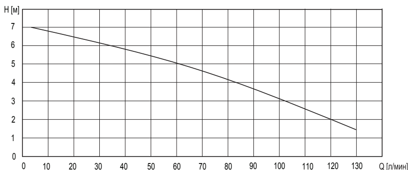
Рис. 1. Гидравлические характеристики.
